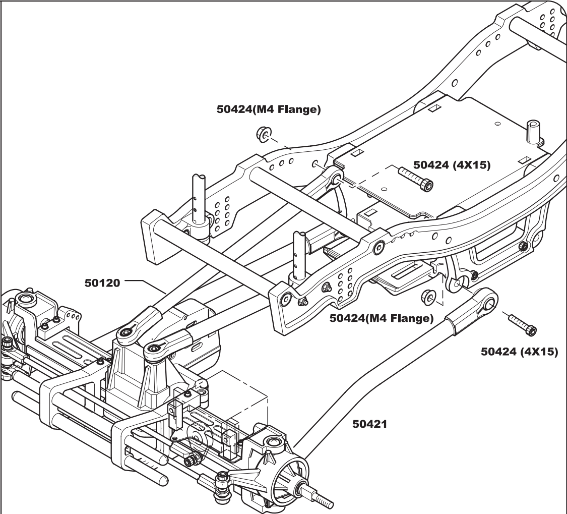
50424(M4 Flange)
